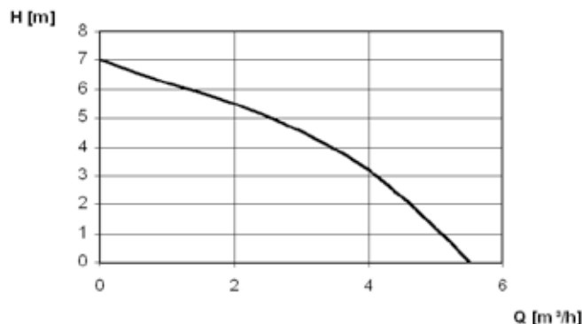
FSP 330 mit elektronischer Niveausteuerng
